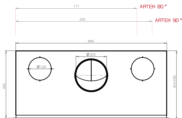
Vista superior
